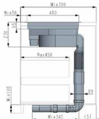
Piano da incasso 700 mm
