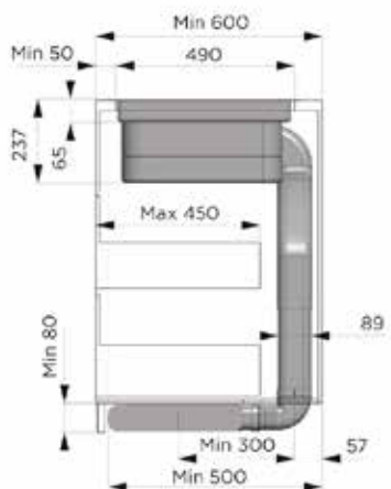
Piano da incasso 600 mm
