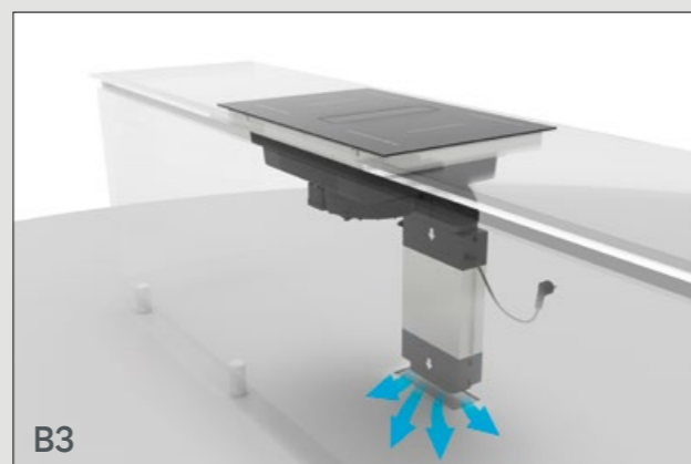
INSTALLAZIONE FILTRANTE CON FILTRO AL PLASMA IN ARIA LIBERA (adatta anche per mobili con piedini)
