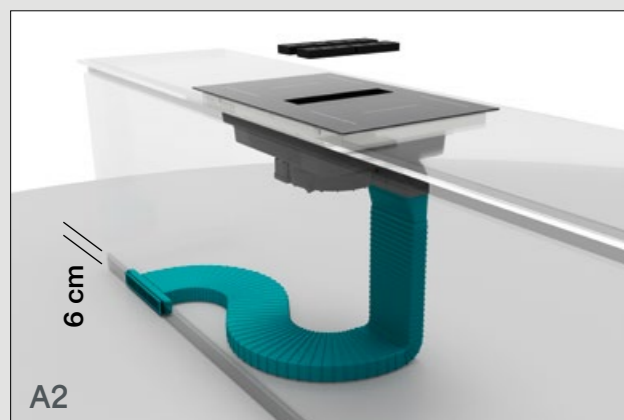
KIT TUBI INSTALLAZIONE FILTRANTE ZOCCOLO H6 cod. 005PRC050001
